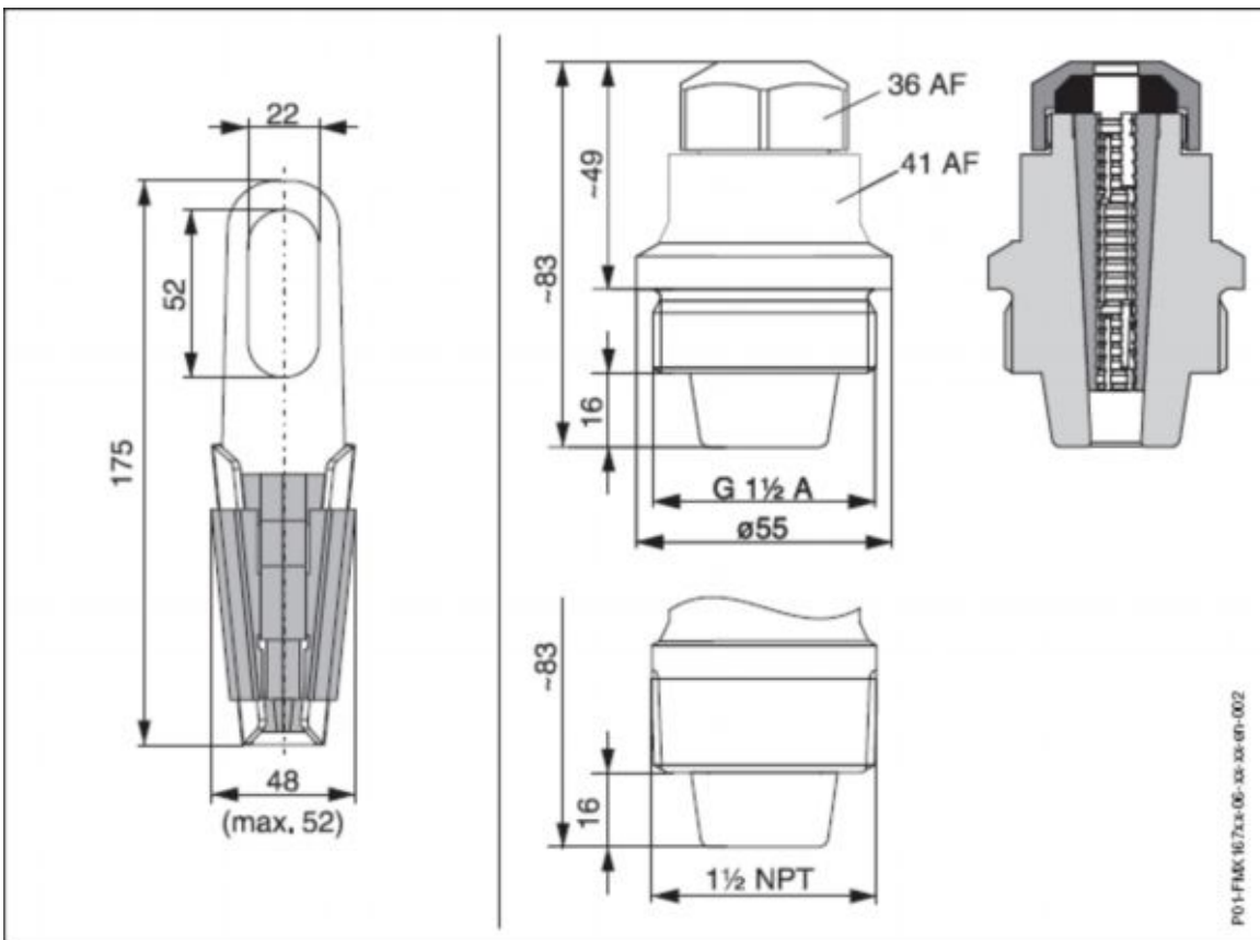
Габариты кабельного уплотнителя 1 ½ NPT FMX 167-□4□□□□□□
