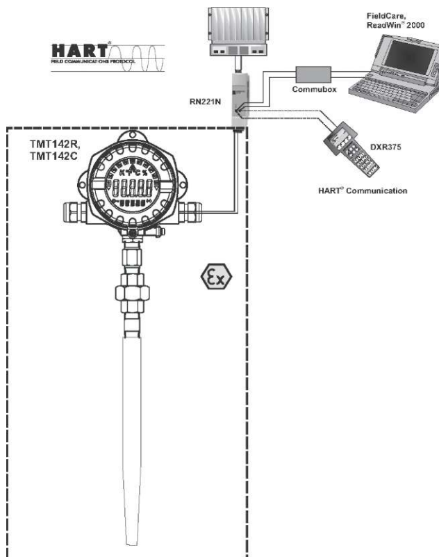
Пример применения компактного термометра
