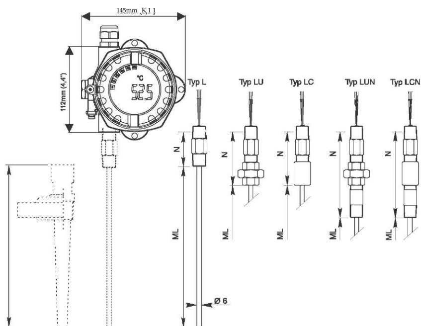
Компоненты датчика
