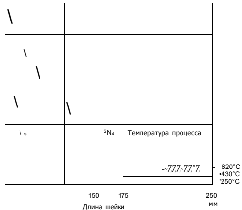
Нагрев головки датчика от в зависимости от длины шейки
